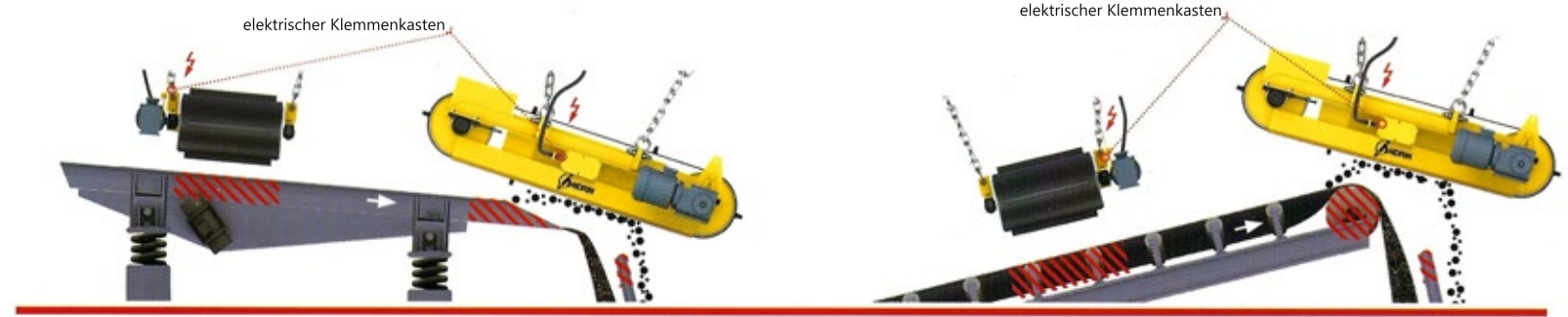
Overband Elektromagneten für Förderer [400 - 2400 mm]
