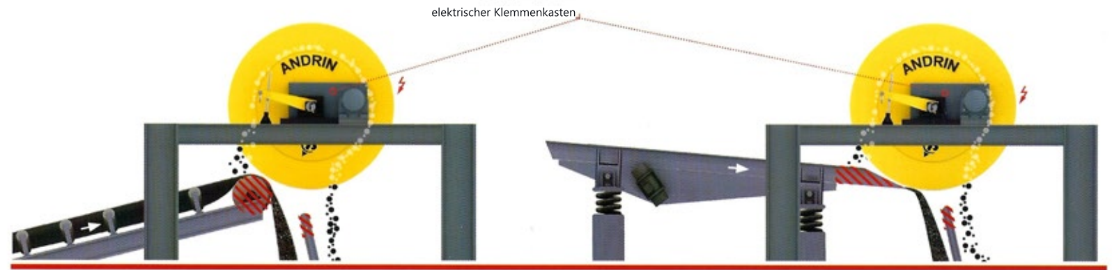
elektromagnetische Trommeln [Ø 320 - 1800 mm / Breite 400 - 3000 mm]
